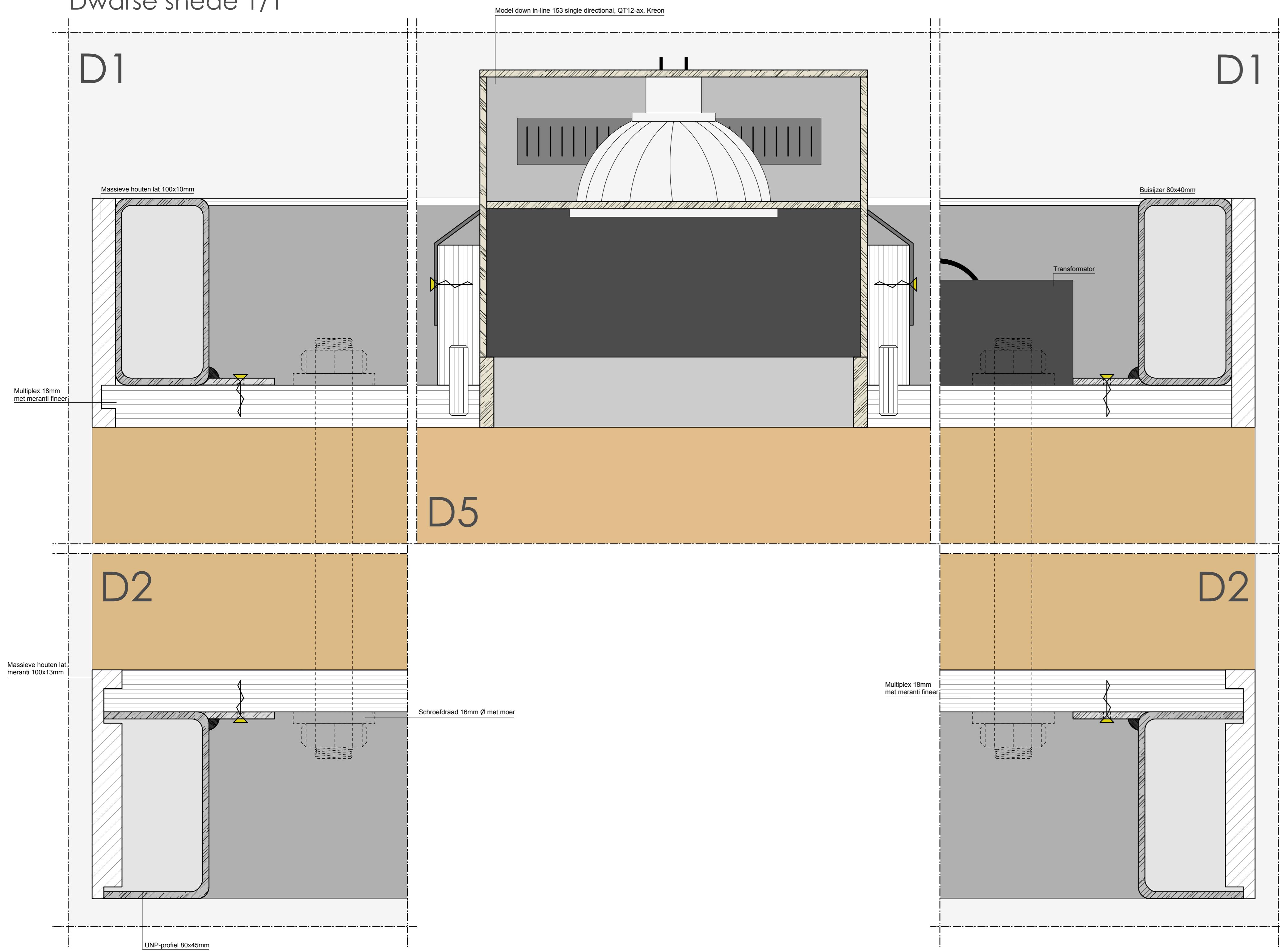
Dwarse snede 1/1
